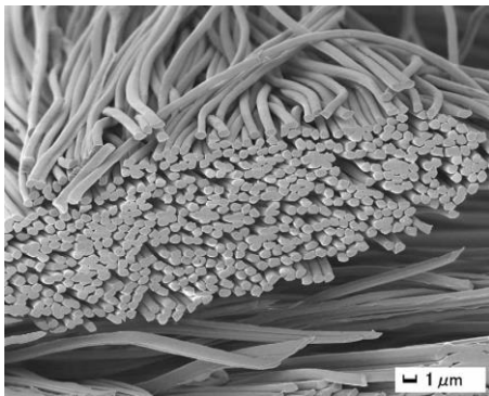
“SOLOTEX®Nanofiber”的截面图
